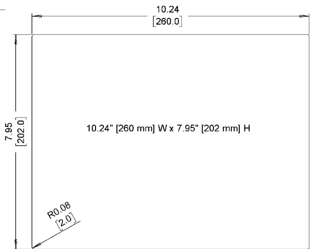
Cutout Dimensions
